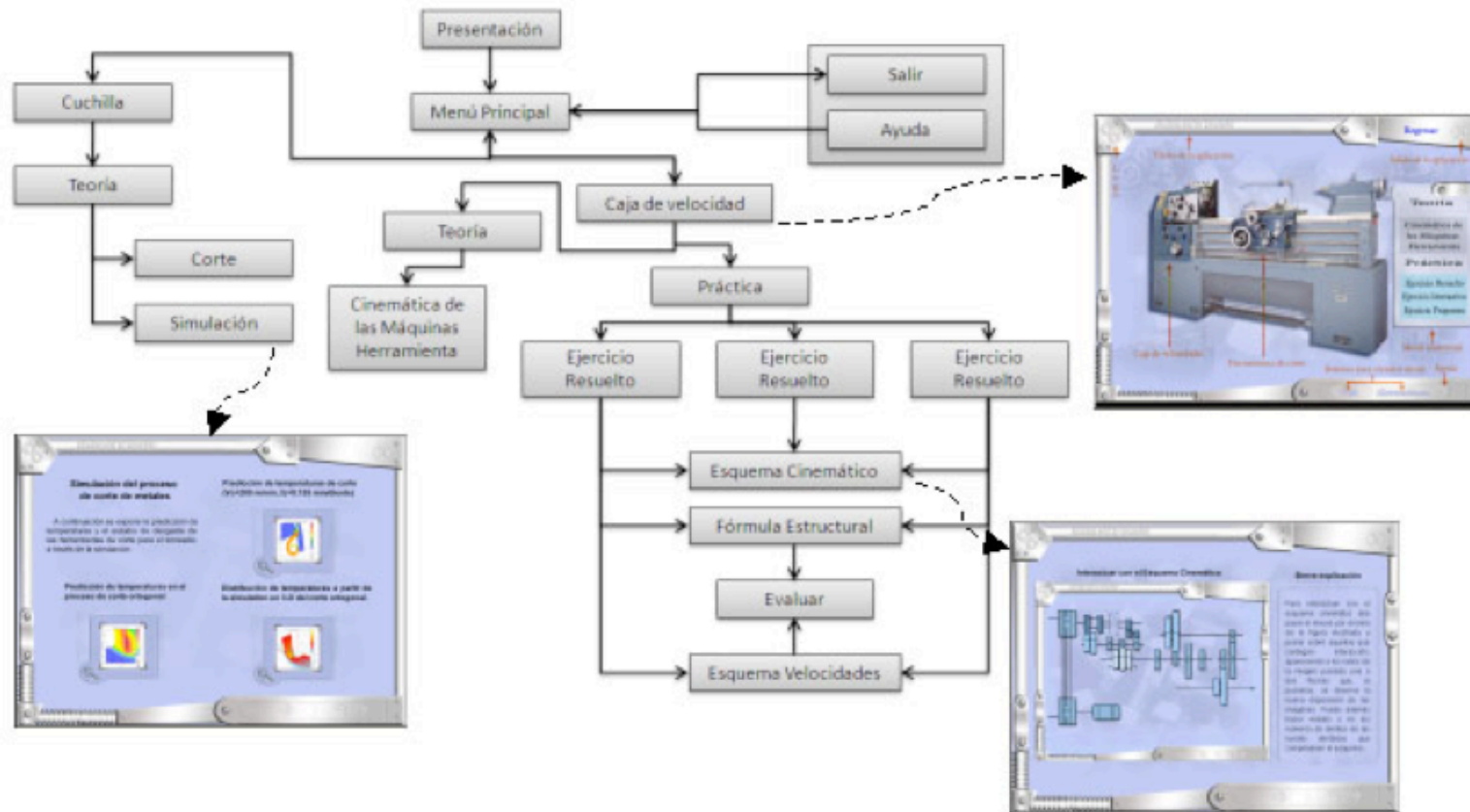
Figura 3. Mapa de navegación de KinMTool.
